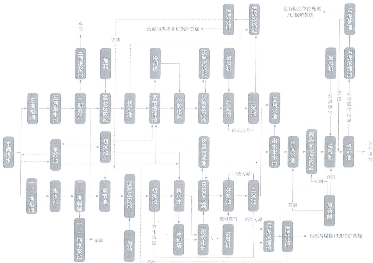
东莞建晖纸业有限公司污水处理系统工艺流程图
