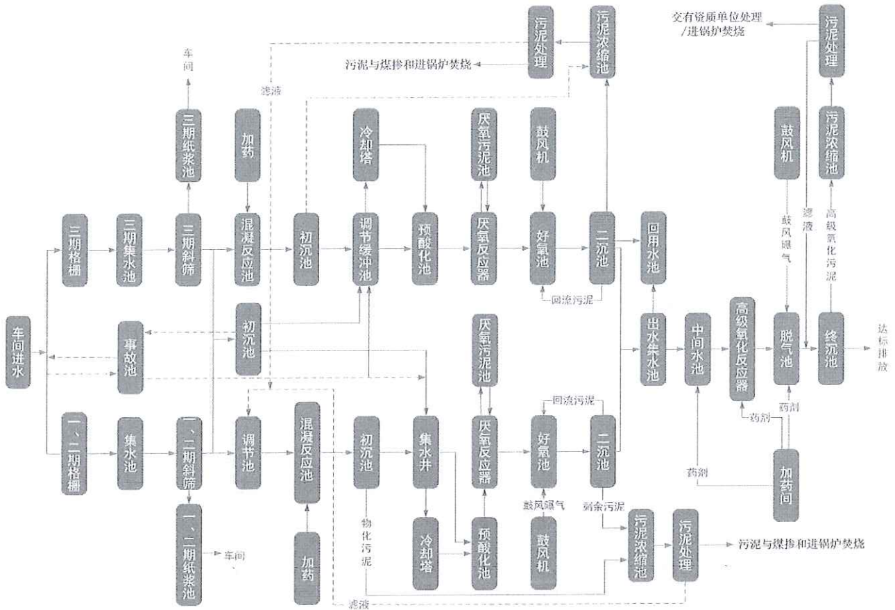
东莞建晖纸业有限公司污水处理系统工艺流程图
